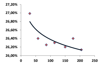
Curva Lebacs
