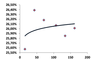
Curva Lebacs
